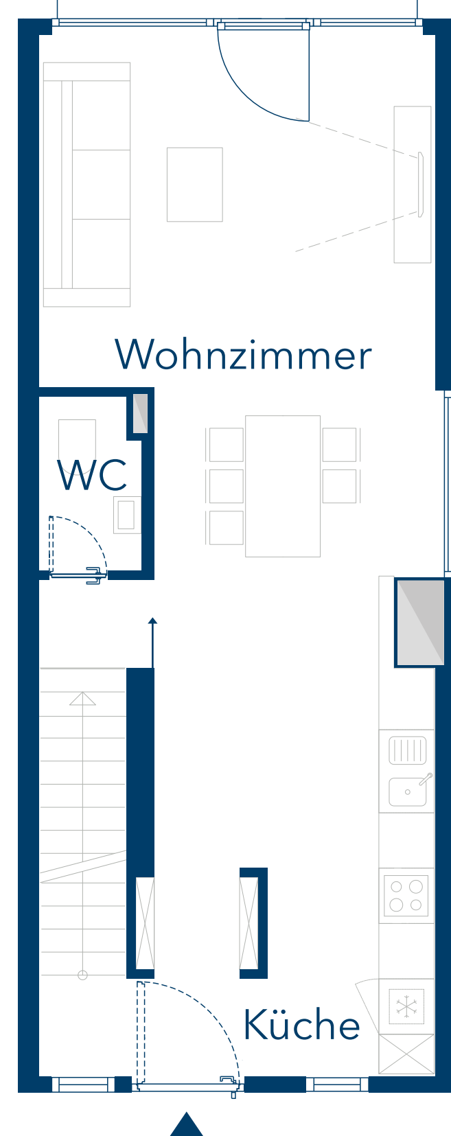
Erdgeschoss
